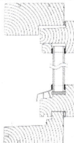
Genomskärning fönsterbäge & karm
